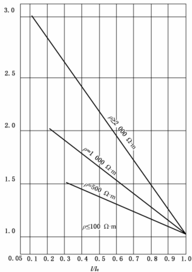
图C.1 换算系数 A
